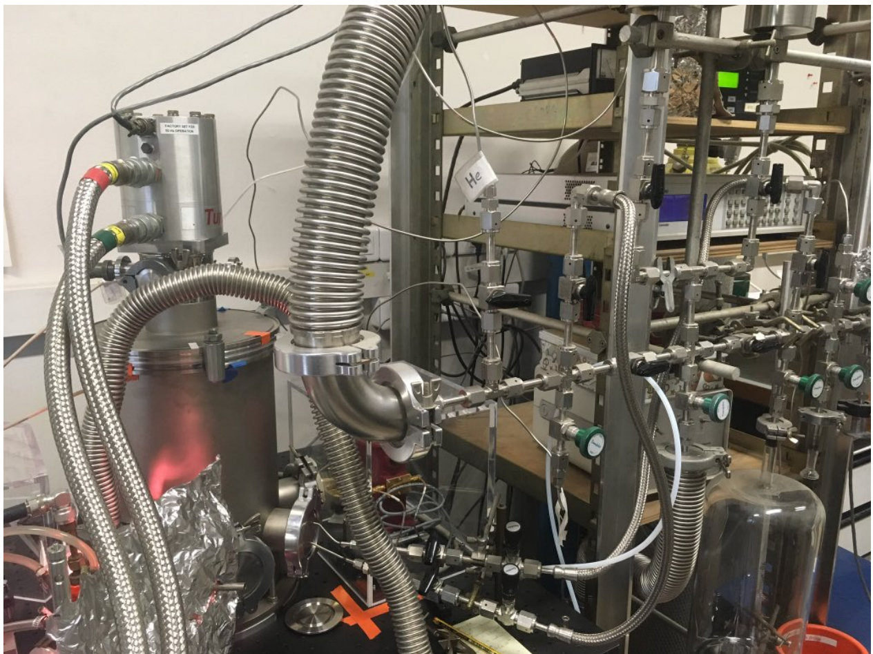
Procédé expérimental de Robin Isnard pour recréer la matière du milieu interstellaire
