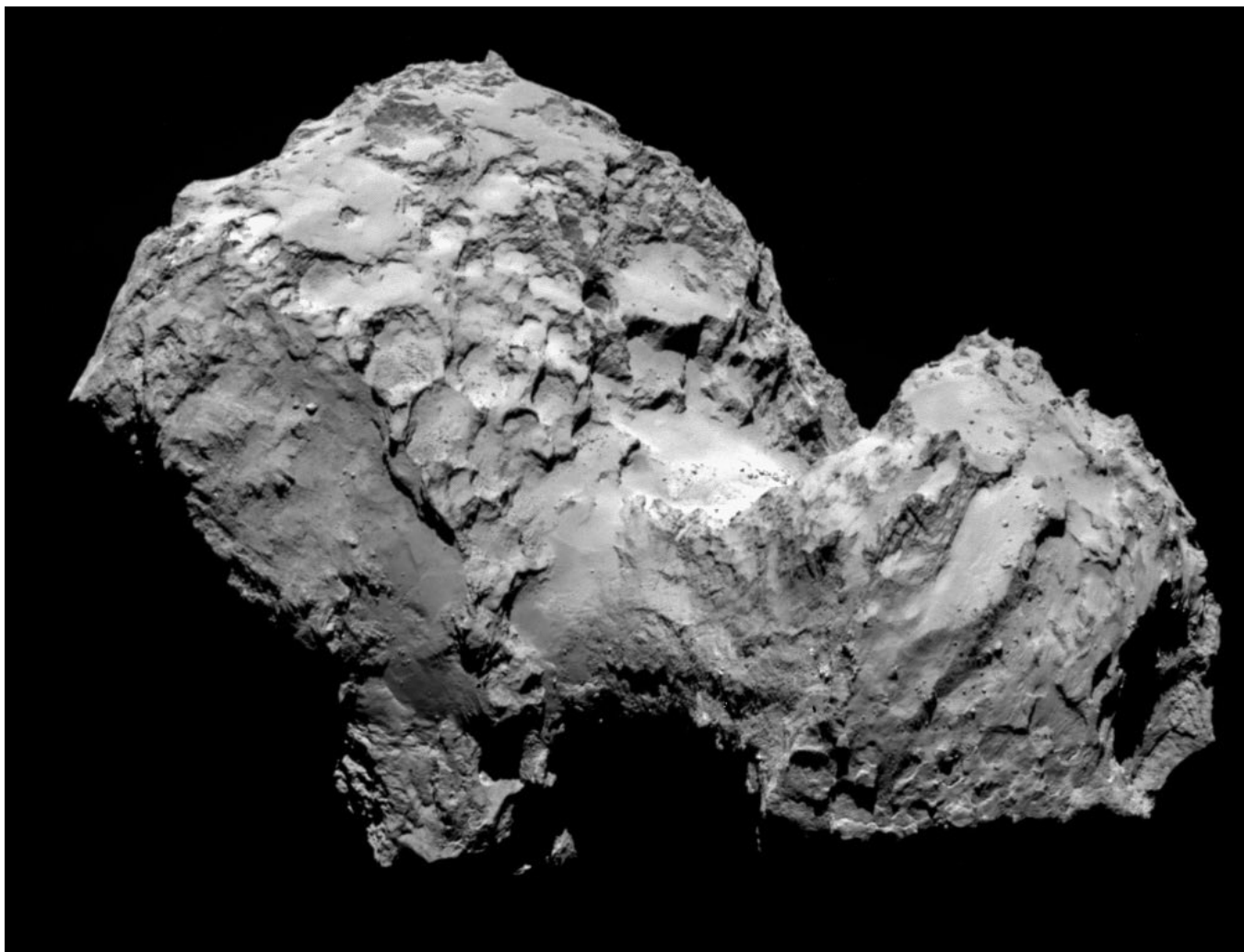
Comète étudiée par la sonde Rosetta : 67P Churyumov gerasimenko
